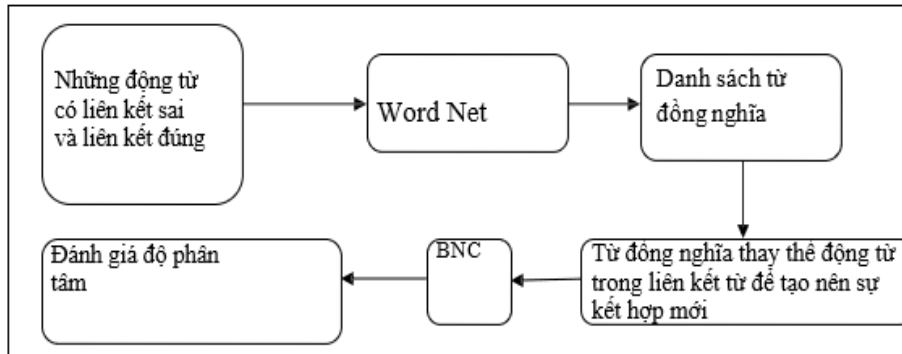
Hình 6. Quá trình tạo yếu tố nhiễu phân tâm trong liên kết từ
